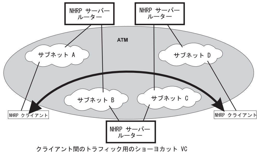
図 27. ネクスト・ホップ解決プロトコル (NHRP) の概要
