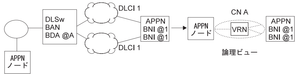
図7. 複数のフレーム・リレー・ポートをもつ BAN を使用する単一の接続ネットワーク
