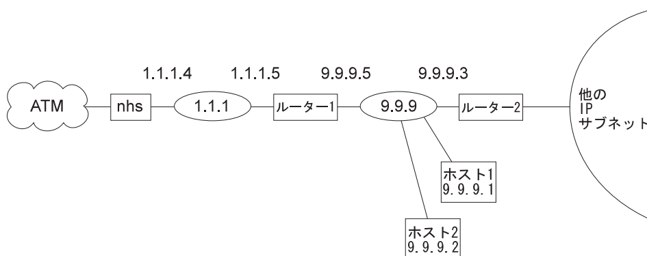
図 34. 不許可ルーター・ツー・ルーター・ショートカットの使用
