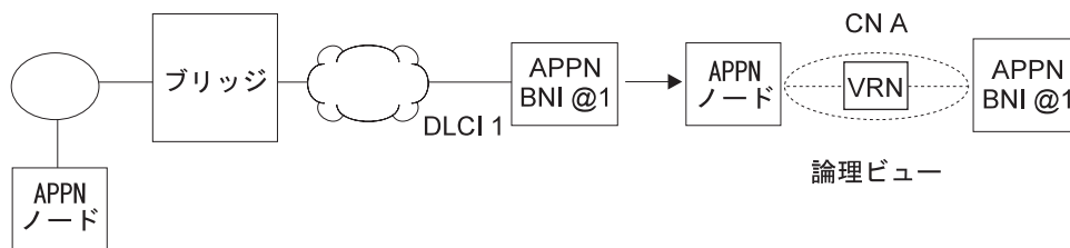
図9. 1つのフレーム・リレー・ポートをもつブリッジングを使用する単一の接続ネットワーク
