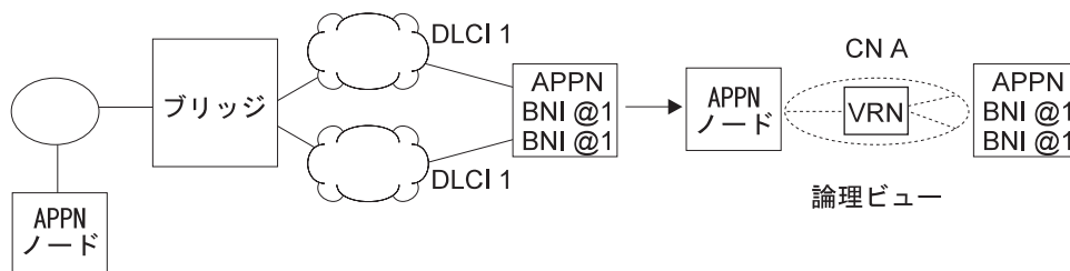
図10. 複数のフレーム・リレー・ポートをもつブリッジングを使用する単一の接続ネットワーク
