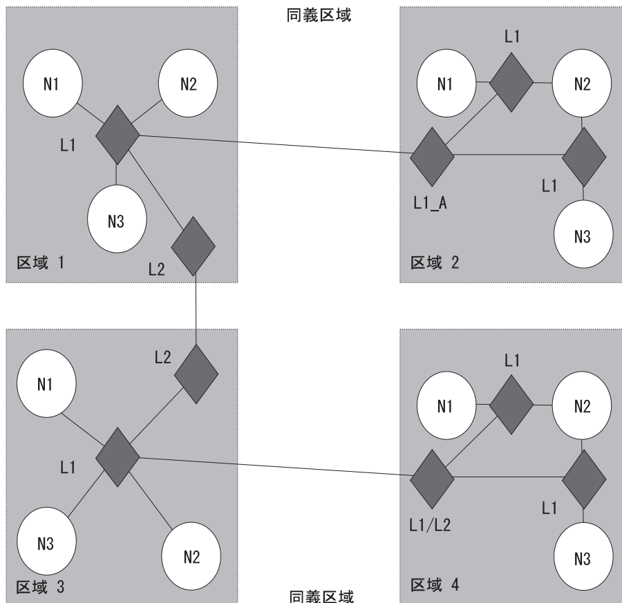
図 25. 同義区域
